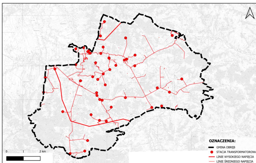
Rys. 14. Linie elektroenergetyczne wysokiego oraz średniego napięcia w gminie Tyczyn.
