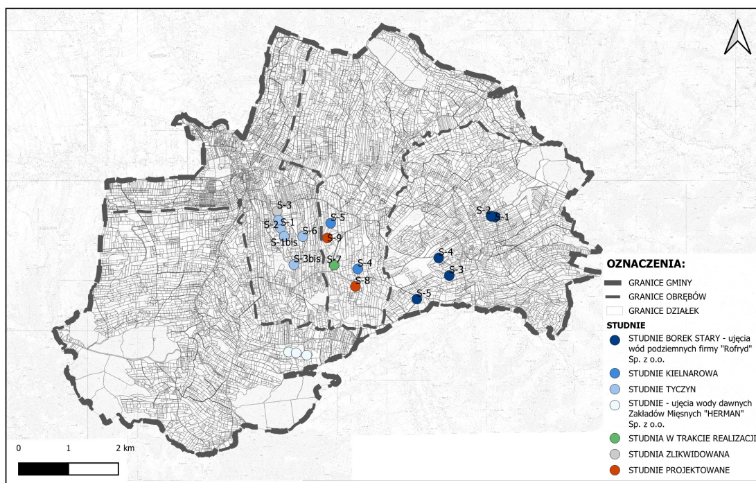
Rys. 6. Lokalizacja ujęć wody dla gminy Tyczyn.
